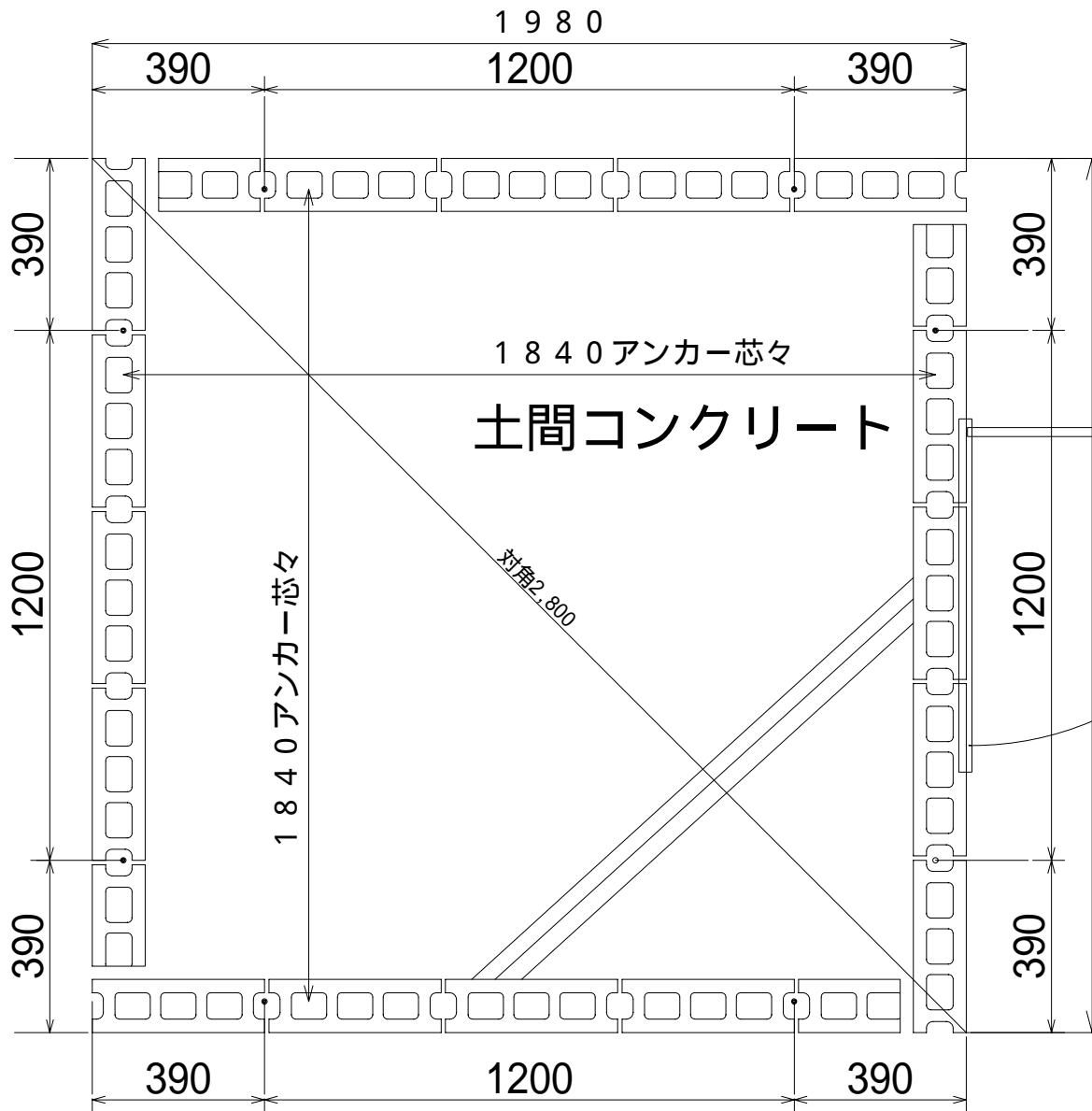
スライドルーフSRL2020 (SRSも同じ) 基礎参考図
