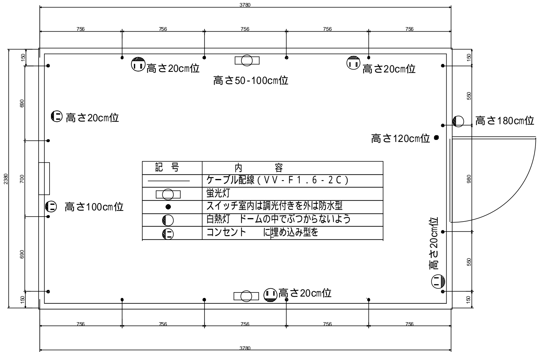
スライドルーフ2400×3800用電気部品配置参考図面
